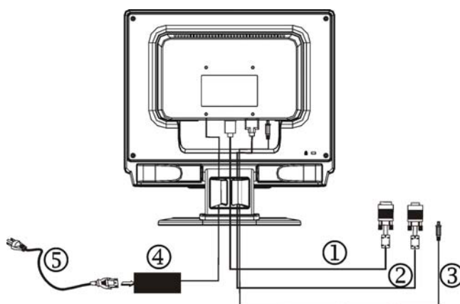
Рис. 1. Подключение кабелей
