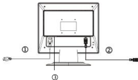
Рис. 1. Подключение кабелей
