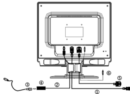
Рис. 1. Подключение кабелей
