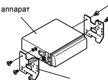
Монтажная рамка
