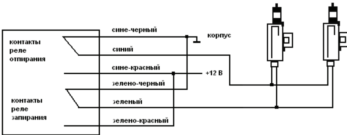
Схема подключения к двухпроводным приводам системы запирания
