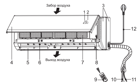
Внутренний блок
