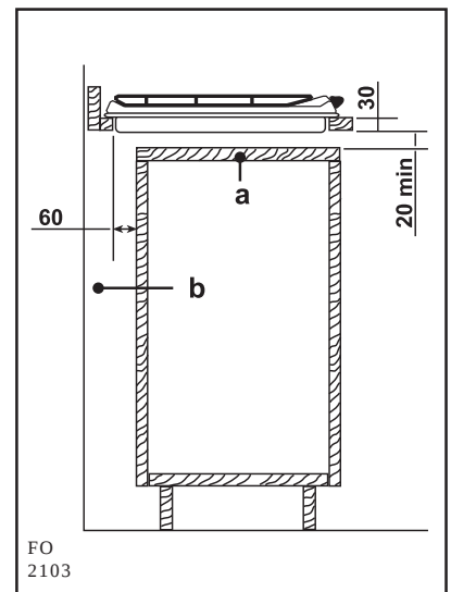
Рис. 11 а) Съемная панель б) Пространство, которое может быть использовано для подключения
