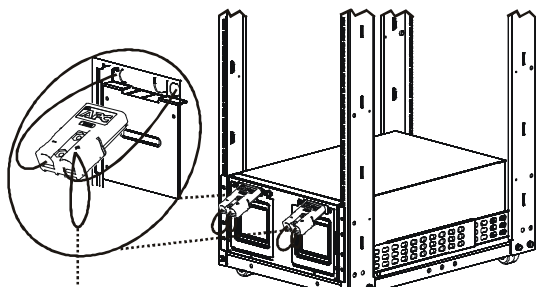
Кабель отключения батарей
