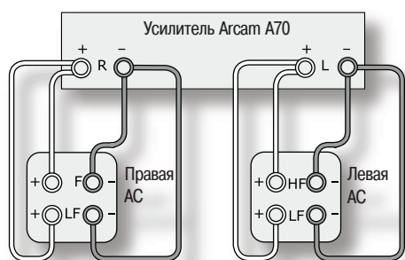
Двухпроводное подключение усилителя
