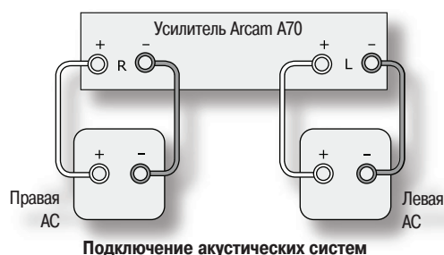
Подключение акустических систем
