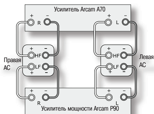
Рекомендованное двухусилительное подключение
