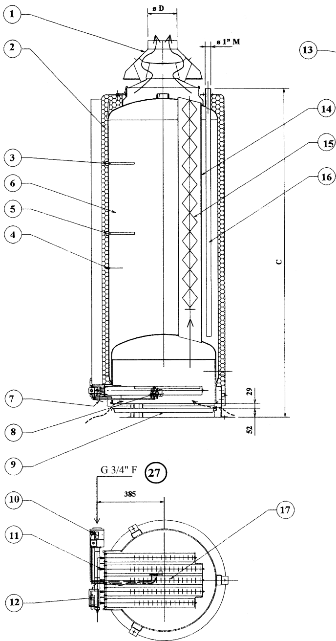
Рис. 3. Схематический разрез
