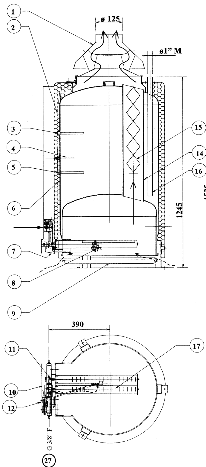
Рис. 1. Схематический разрез
