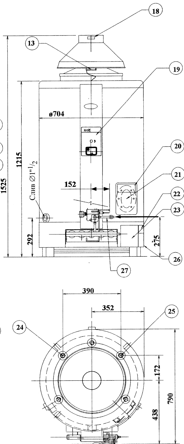
Рис. 2. Габаритные размеры
