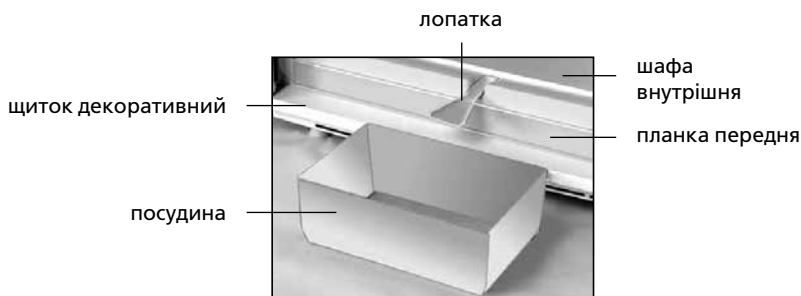
Рисунок 5 – Збір талої води
