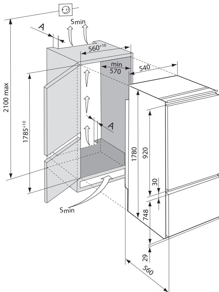
Рисунок 7 – Схема установки холодильника в мебели
