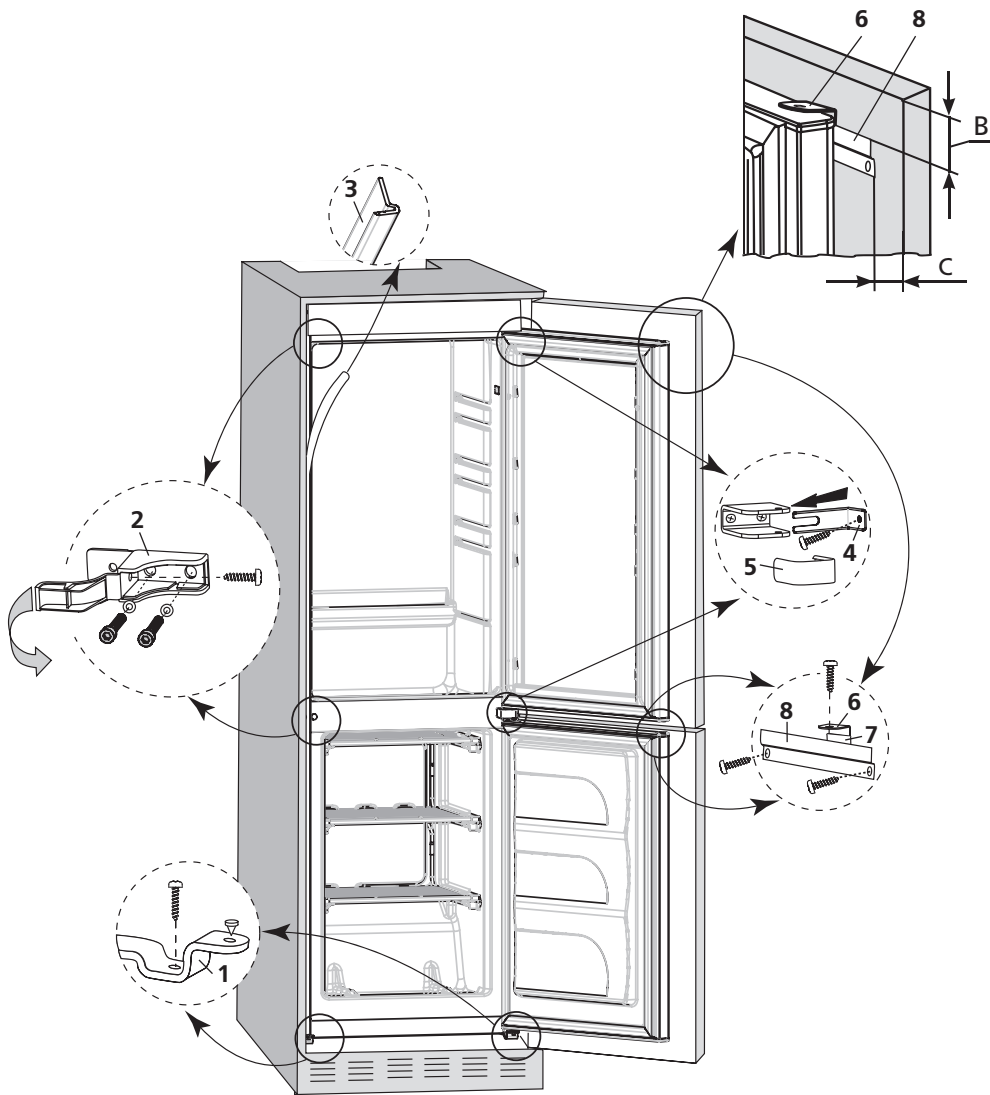
Расми 9 – Нақшаи мустаъкам кардани яхдони дохили мебел
