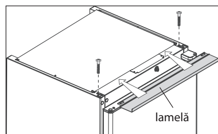
Figura 8 – Instalarea lamelei
