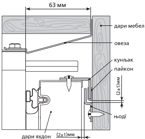
Расми 10 – Нақшаи васли дарёи яхдон ва мебел
