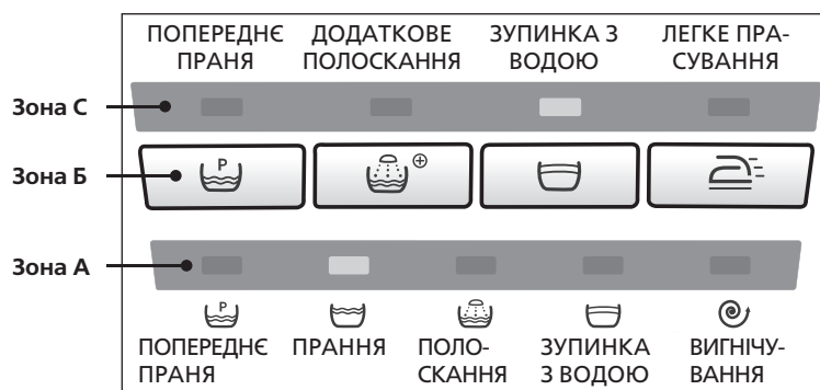
Зона А — індикатори операцій прання; Зона Б — кнопки вибору додаткових функцій; Зона С — індикатори додаткових функцій
