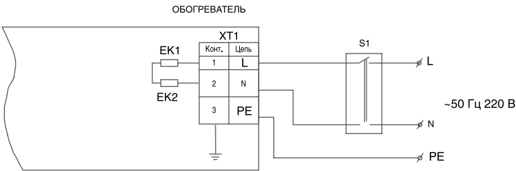
Рис. 2. Обогреватель BIH-APL-2.0
