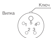
Рис. 5. Схема подключения контактов на вилку (ВНР-9.000, ВНР-15.000)
