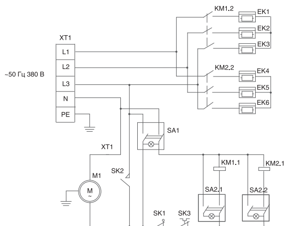
Рис. 6. Схема электрическая тепловентиляторов ВНП-24.000, ВНП-30.000
