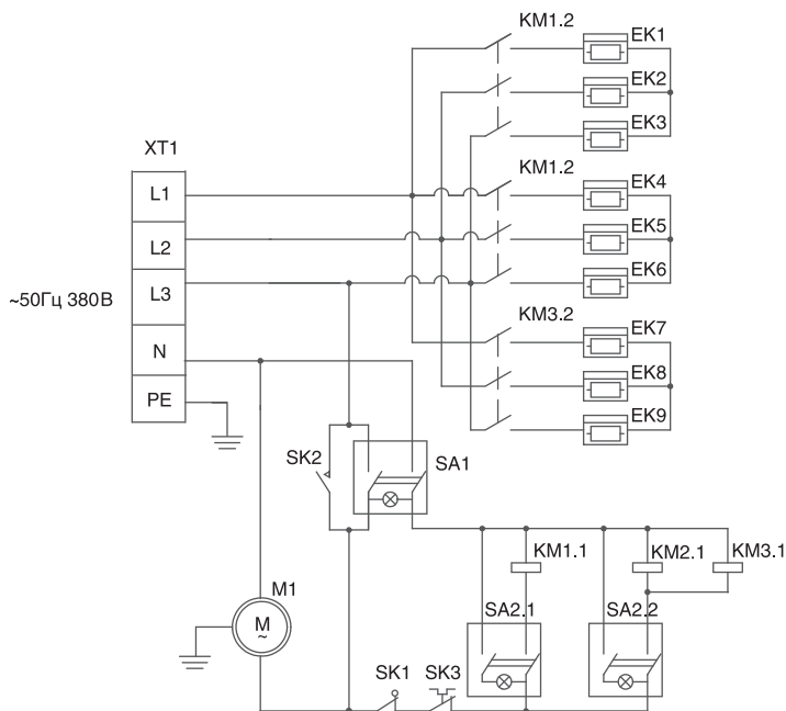
Рис. 6. Схема электрическая тепловентиляторов ВНП-24.000, ВНП-30.000
