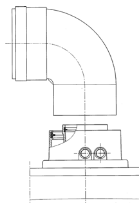
Коаксиальная выходная муфта
