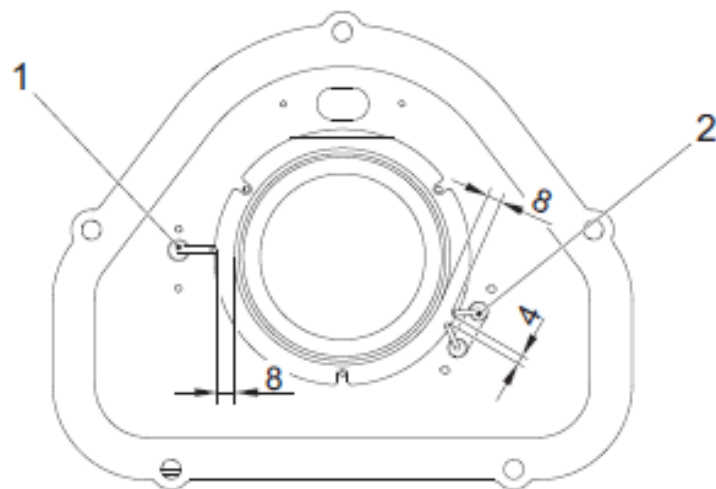
Рис. 39: Расстояния между электродами и монтажные положения
