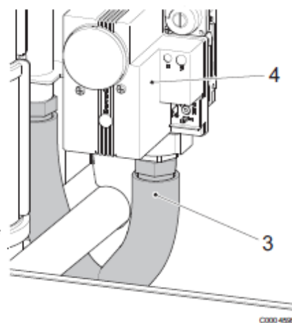
Fig. 35: Вытащить шланг подключения газа из газового клапана
