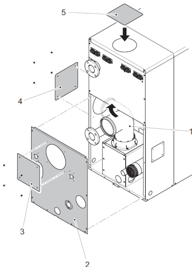
Рисунок 3. Изменение соединений для отвода газов и подачи воздуха
