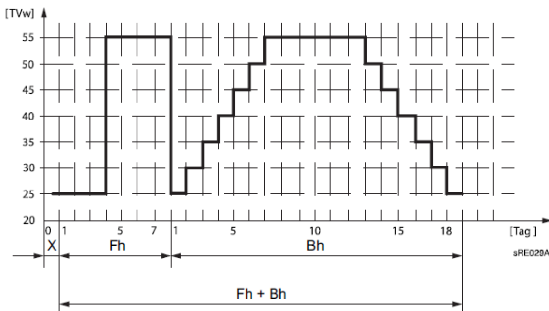
Рис. 21 Контур температуры в режиме высыхания стяжки
