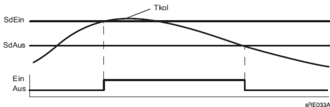
Рис.26 Регулятор загрузки (dT)
