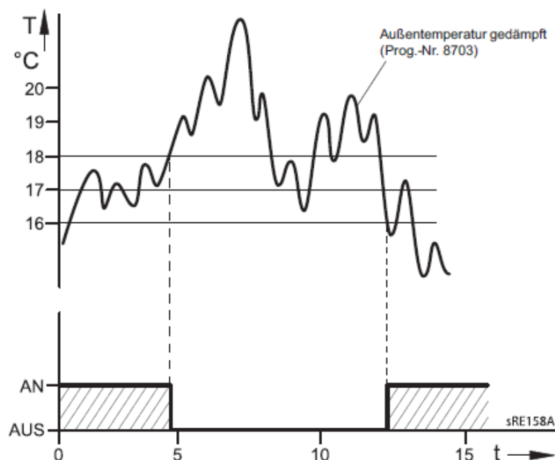
Рис.16 Предельная величина лето/зима
