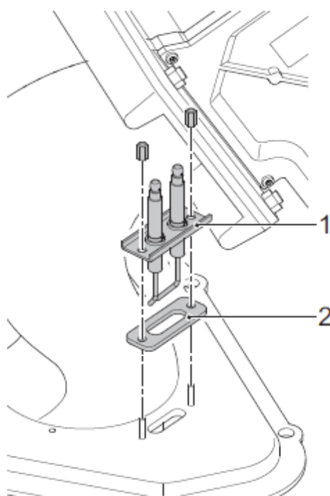
Рис. 37: Демонтаж блока электродов зажигания
