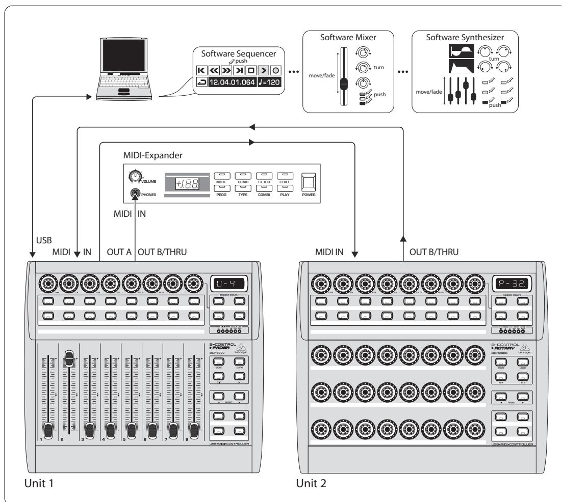
Рис. 4.4: Использование в режиме USB 4 (Expanded)
