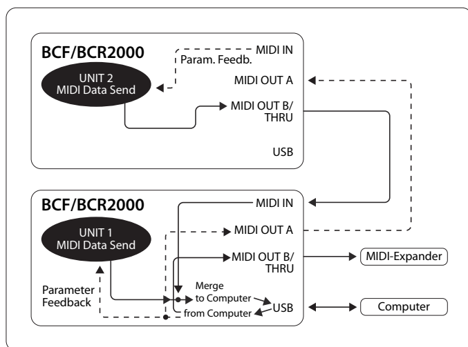
Рис. 4.5: Маршрутизация в режиме USB 4
