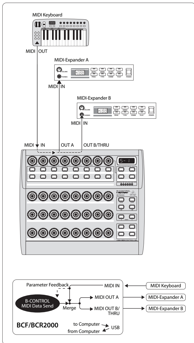
Рис. 4.6: Использование и маршрутизация в автономном режиме 1
