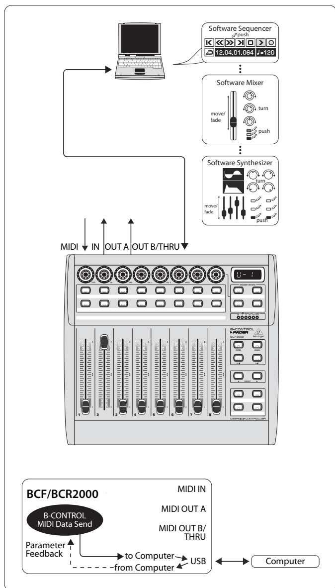
Рис. 4.1: Маршрутизация и использование в режиме USB 1
