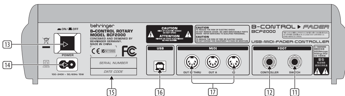
Рис. 3.2: Задняя панель BCF2000 (элементы управления с 13 по 17 совпадают с аналогичными элементами BCR2000)
