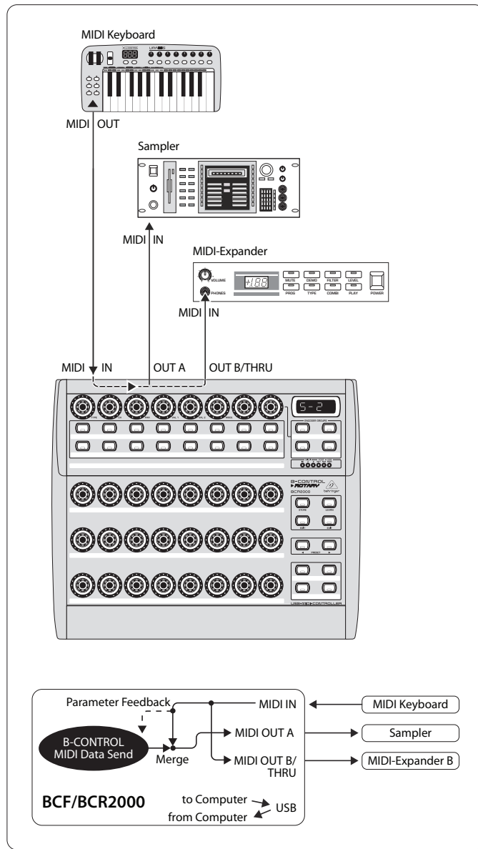
Рис. 4.7: Использование и маршрутизация в автономном режиме 2
