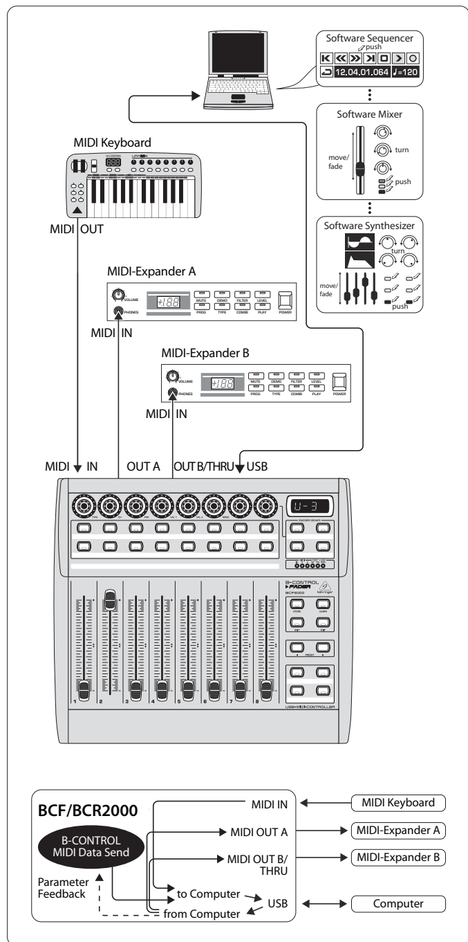
Рис. 4.3: Маршрутизация и использование в режиме USB 3
