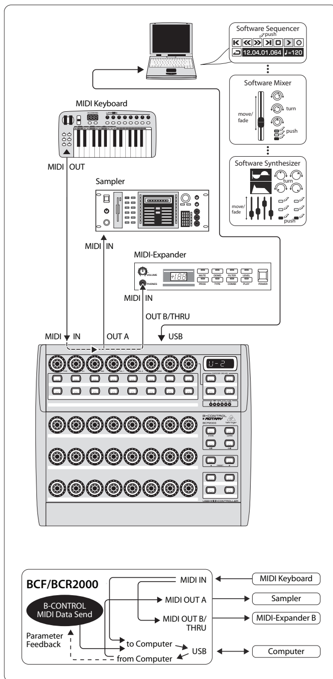
Рис. 4.2: Маршрутизация и использование в режиме USB 2
