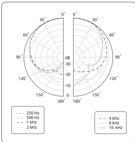
Полярная диаграмма
