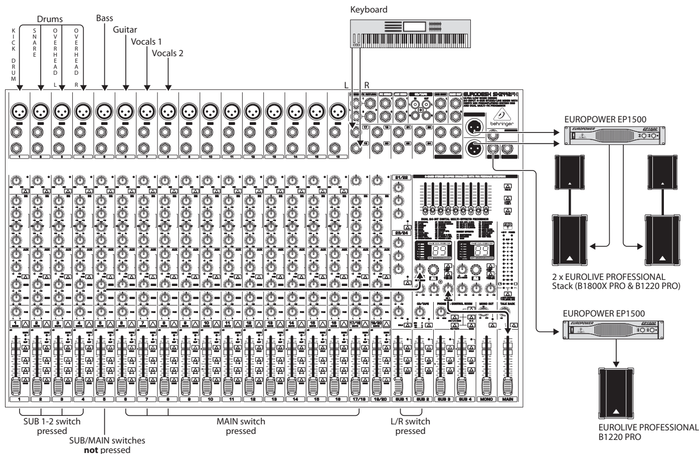
Рис. 4.2: Подключение микшерного пульта для работы на сцене
