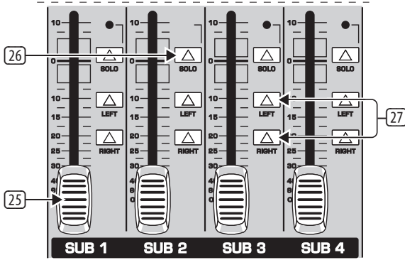
Рис. 2.9: Подгруппы 1-4
