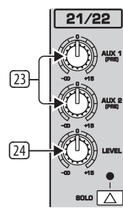
Рис. 2.8: Дополнительные стереоканалы
