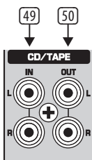
Рис. 2.21: Разъемы CD/Tape
