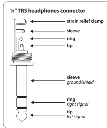
Рис. 5.6: Стереоштекер наушников
