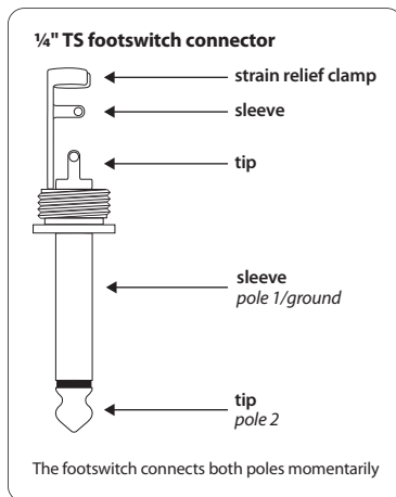
Рис. 5.5: Стереоштекер педального выключателя
