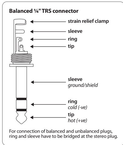
Рис. 5.2: 6,3-мм TRS-штекер
