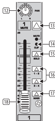
Рис. 2.4: Канальный фейдер, регулятор Pan, выключатель Mute и др.
