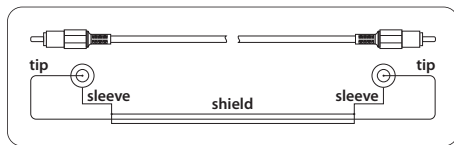
Рис. 5.3: Cinch-кабель
