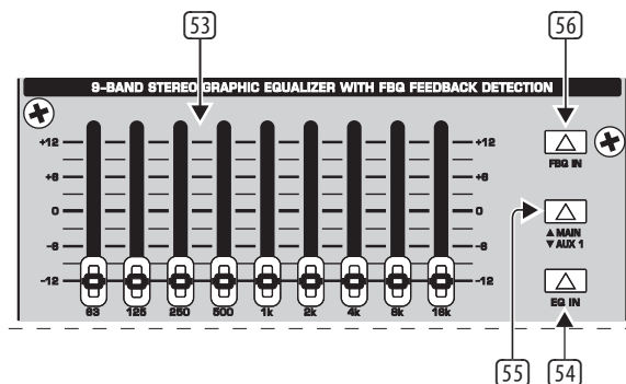
Рис. 2.24: Графический стереоэквалайзер
