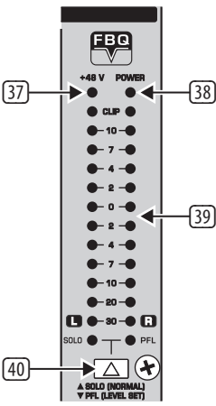
Рис. 2.16: Индикация уровня
