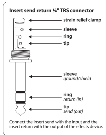
Рис. 5.7: Стереоштекер Insert-Send-Return
