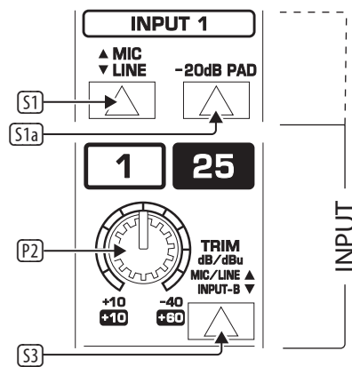
Fig. 3.1: Input
