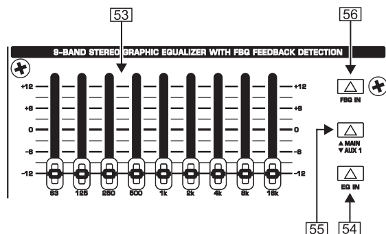
Рис. 2.24: Графический стереоэквалайзер
