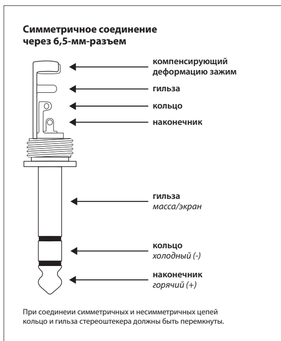
Рис. 5.2: 6,3-мм TRS-штекер
