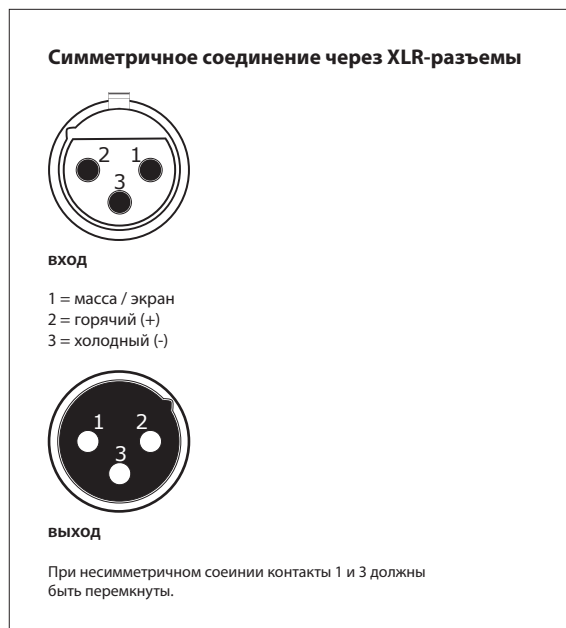
Рис. 5.4: Разъемы XLR
