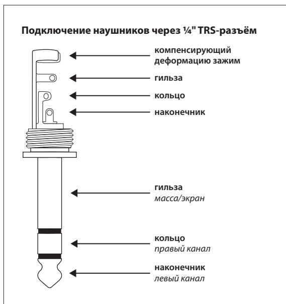
Рис. 5.6: Стереотекек наушников
