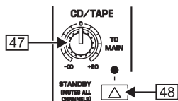
Рис. 2.20: CD/Tape
