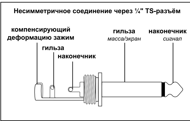
Рис. 6.2: 6,3-мм моноштекер
