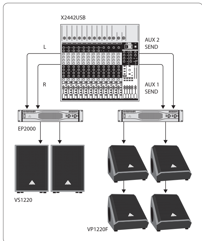
Фиг. 5.2: Стерефонический режим с полным частотным диапазоном и напольными мониторами
