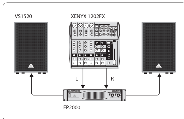
Фиг. 5.1: Стерефонический режим с полным частотным диапазоном
