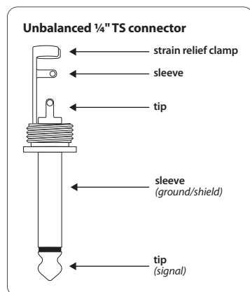
Фиг. 2.2: Разъем TS для громкоговорителей размером ¼ дюйма
