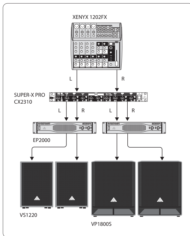
Фиг. 5.3: Двухканальный стереофонический режим с сабвуферами
