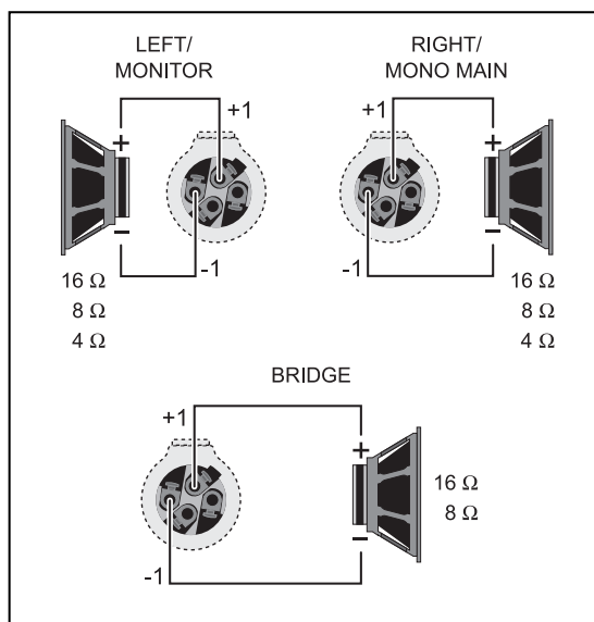
Рисунок 4.6: Спикер-штекер и его распиновка
