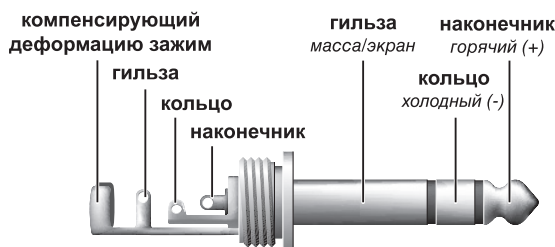
Рисунок 4.2: 6,3-мм-стереоштекер
