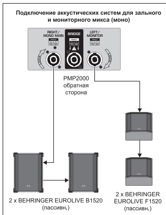
Рисунок 5.2: PMP2000 в качестве двойного моноусилителя (пример)
