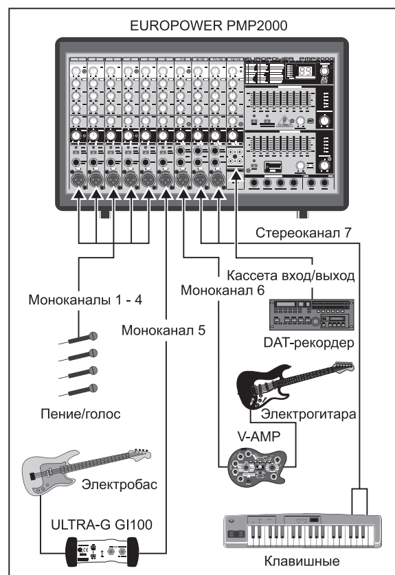
Рисунок 5.3: Стандартное исполнение (пример)
