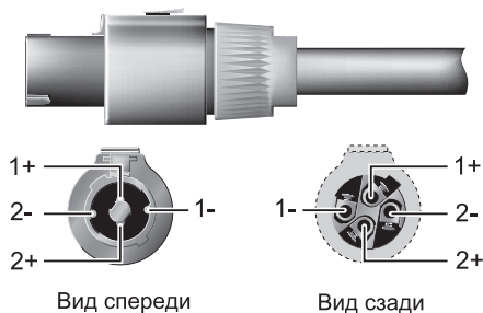
Рисунок 4.5: Профессиональное подключение акустических систем
