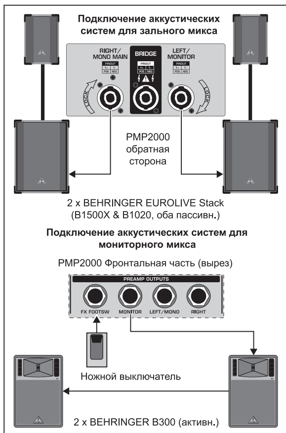
Рисунок 5.1: PMP2000 в качестве стереоусилителя (пример)
