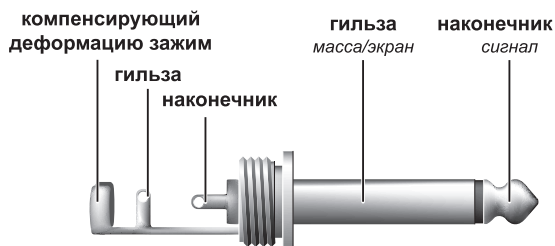
Рисунок 4.1: 6,3-мм-моноштекер
