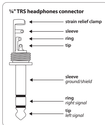
Рис. 4.4: Стерефонический штекер наушников
