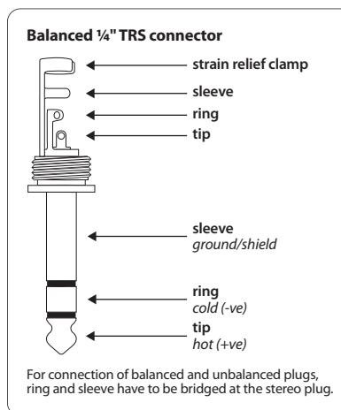
Рис. 4.3: Стерефонический штекер 6,3 мм
