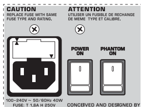
Рис. 2.16: Поддача питания и предохранитель
