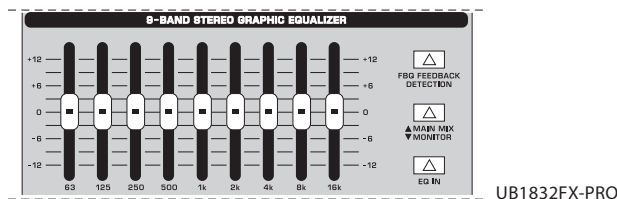
Рис. 3.1: Графический стереоэквалайзер пульта UB1832FX-PRO
