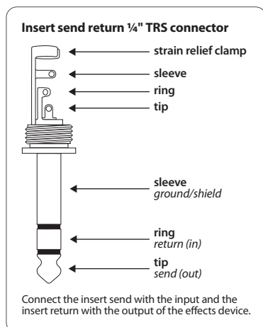
Рис. 6.5: Стереостекер „Insert-Send-Return“
