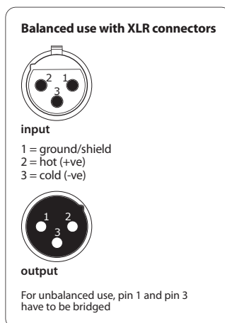
Рис. 6.2: Соединения XLR
