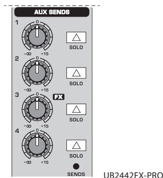
Рис. 2.7: Регуляторы посыла AUX SEND основной секции
