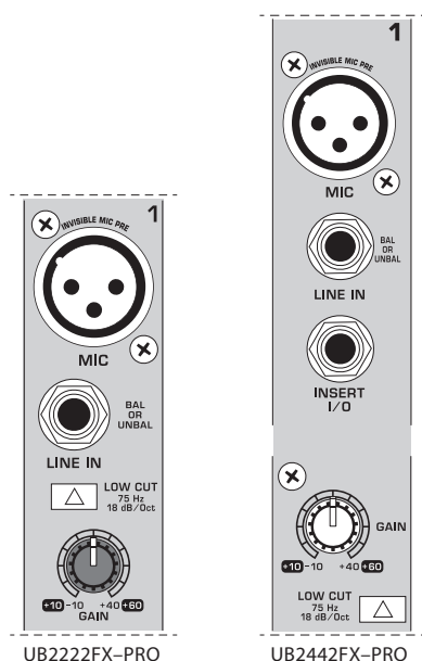
Рис. 2.1: Разъёмы и регуляторы микрофонных и линейных входов
