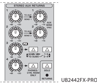
Рис. 2.12: Регуляторы Stereo Aux Return и Stereo Aux Return (to Aux Send)
