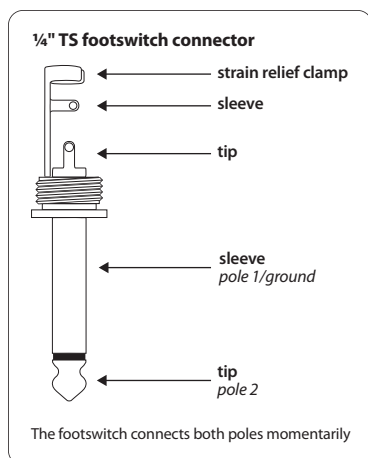
Рис. 6.1: Штекер педального выключателя
