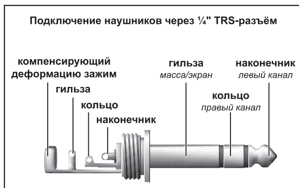
Рис. 6.6: Стереоштекер наушников
