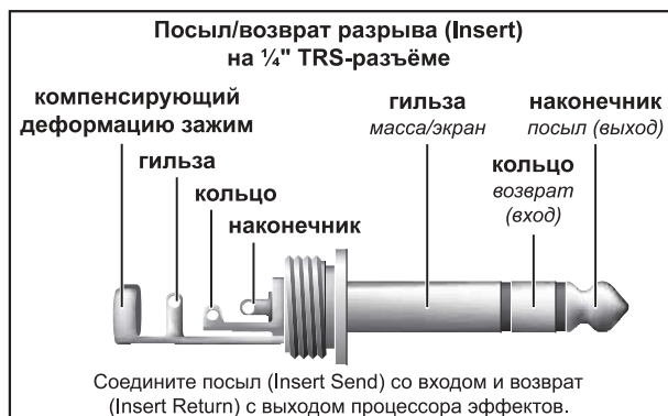
Рис. 6.5: Стереоштекер „Insert-Send-Return“
