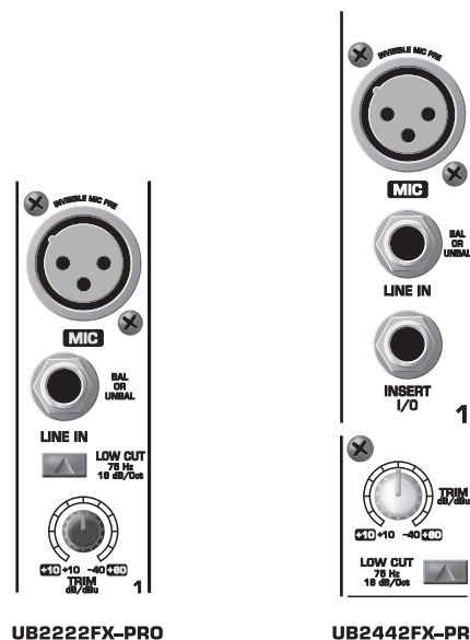
Рис. 2.1: Разъёмы и регуляторы микрофонных и линейных входов
