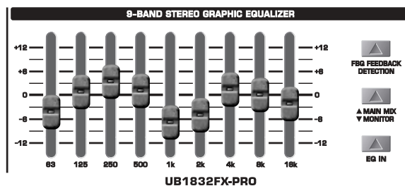
Рис. 3.1: Графический стереоэквалайзер пульта UB1832FX-PRO
