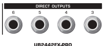
Рис. 5.4: Прямые выходы
