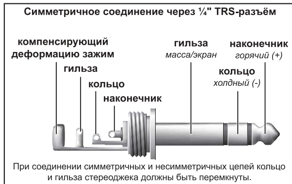
Рис. 6.4: Стереоштекер 6,3 мм
