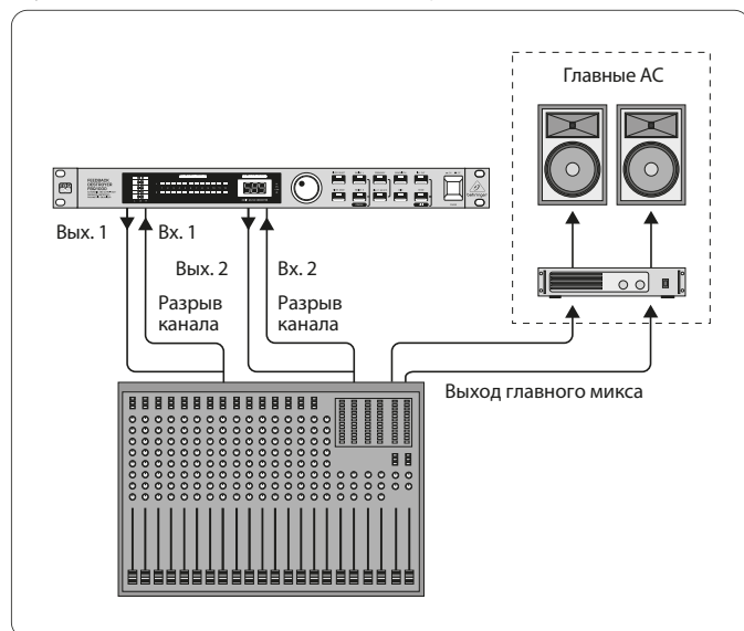
Рисунок 2.2: Использование FBQ1000 для отдельных микрофонов (включение подавителя обратной связи в разрыв канала или подгруппы)
