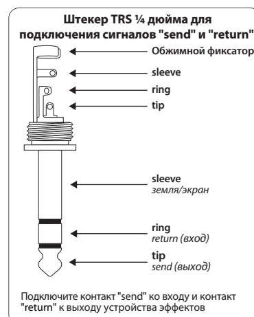
Рисунок 10.1: Подключение кабеля "INSERT" (для включения устройства в разрыв канала)
