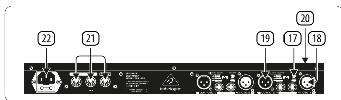
Рисунок 4.3: Разъемы и элементы управления на задней панели
