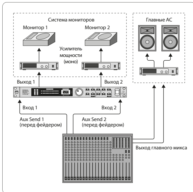
Рисунок 2.1: Использование FBQ1000 в каналах мониторов
