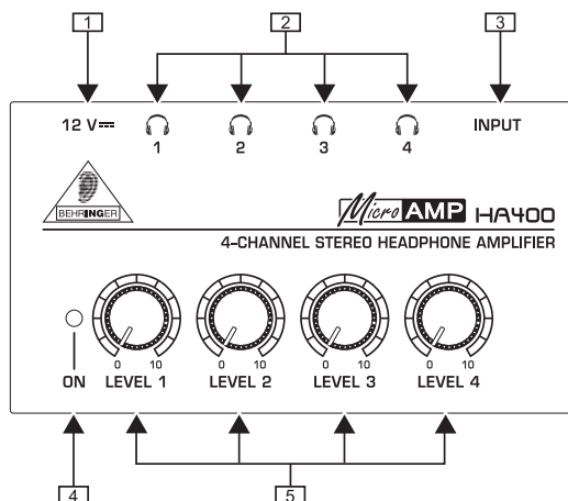
Элементы управления и присоединение HA400
