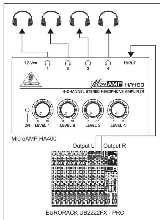
Каблирование HA400
