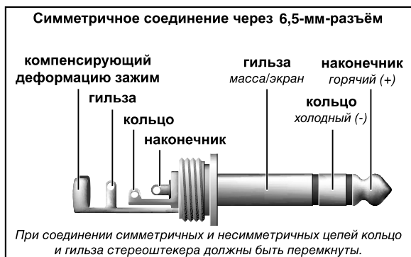
Рисунок 5.2: 6,5-мм-стереоштекер
