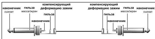
Рис. 5.1: Разводка инструментального кабеля
