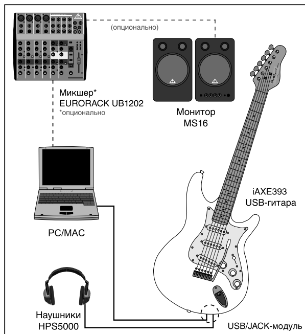
Рис. 4.1: Подключение USB-гитары
