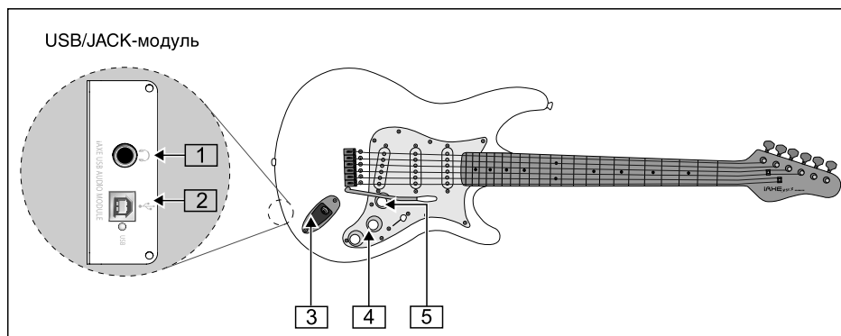
Рис. 2.1: Элементы управления и разъемы
