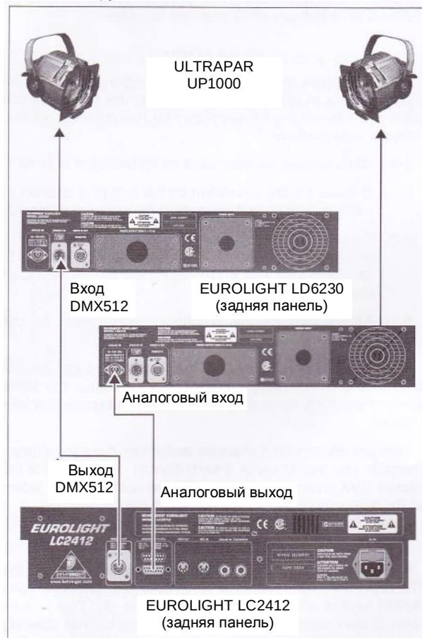
Рисунок 3.1: Пример подключения с пультом EUROLIGHT LC2412 и прожекторами ULTRAPAR UP1000
