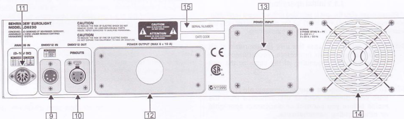
Рисунок 2.2: задняя панель блока EUROLIGHT LD6230
