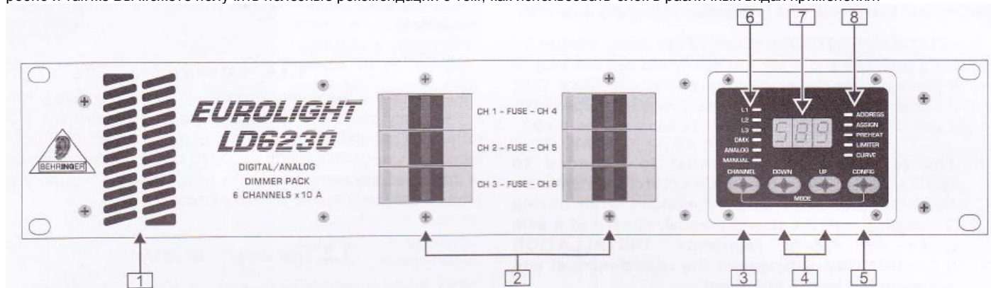
Рисунок 2.1: передняя панель блока EUROLIGHT LD6230
