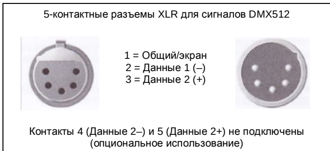
Рисунок 4.1: Назначение выводов 5-контактного разъема XLR
