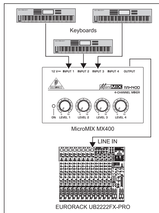
Каблирование MX400
