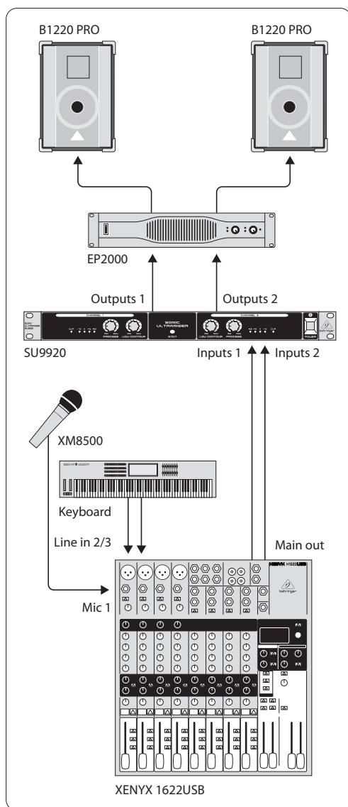
Рис. 3.1: Работа SU9920 с системами озвучения
