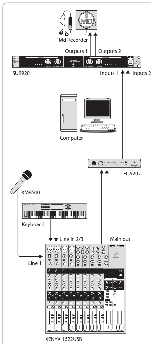
Рис. 3.2: Работа с SU9920 в студии
