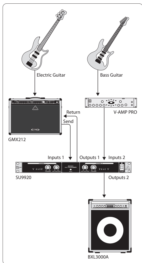
Рис. 3.3: Работа SU9920 с гитарными усилителями
