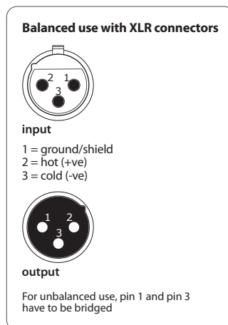
Рис 4.3: Симметричный XLR-штекер
