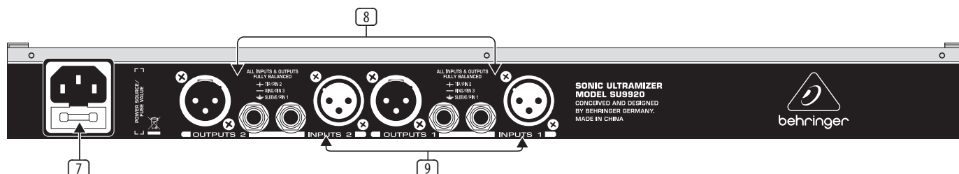
Рис. 2.2: Задняя панель, элементы управления
