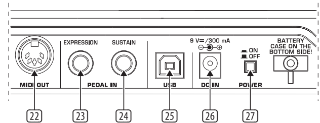
Рис. 3.3: Другие соединения на задней панели
