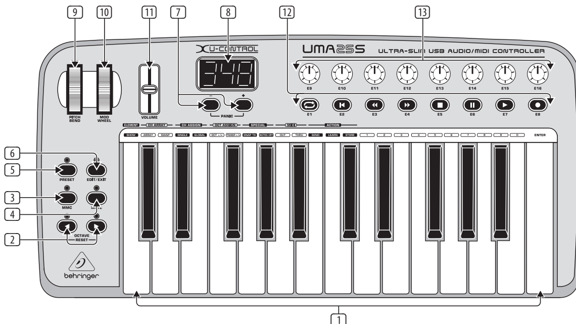
Рис. 3.1: Панель управления U-CONTROL
