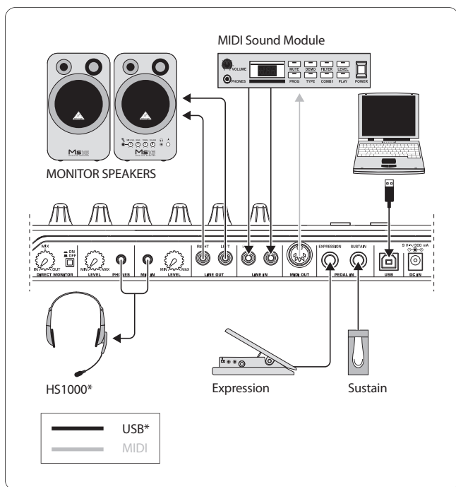
* входит в комплект поставки Рис. 1.3: Пример соединения
