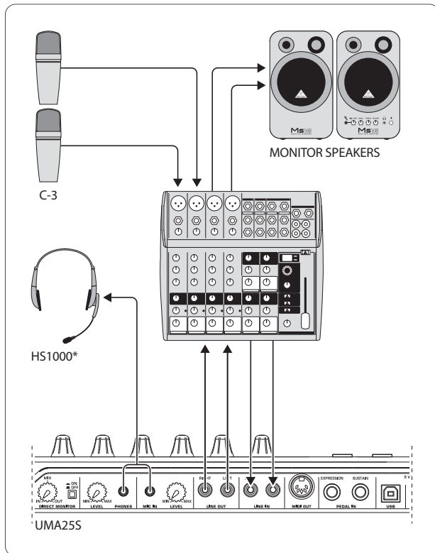
Рис. 4.1: Пример использования UMA25S
