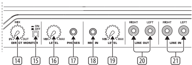
Рис. 3.2: Аудиосоединения на задней панели
