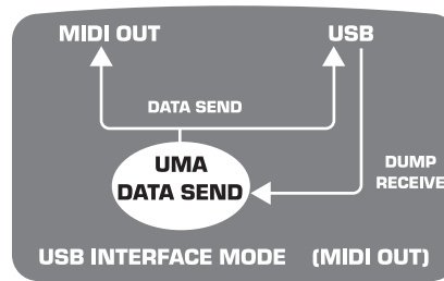
Рис. 1.6: Режим USB с MIDI OUT
