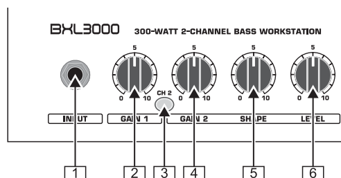
Рис. 2.1: Входная секция
