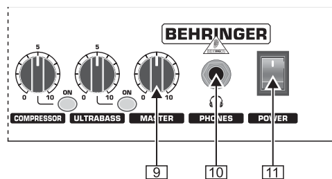
Рис. 2.3: Мастер-секция
