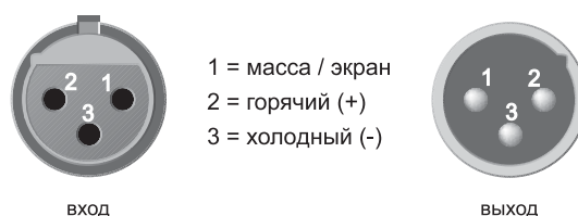
Рис. 5.1: Разъемы XLR
