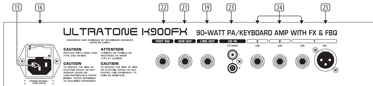
Рис. 2.4: Элементы управления задней панели (K900FX и K450FX)
