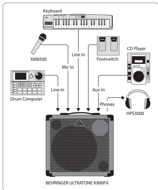
Рис. 3.1: Пример устройства, подключенного к ULTRATONE
