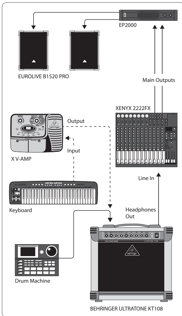
Рис. 2.2: Установка для “живых” выступлений
