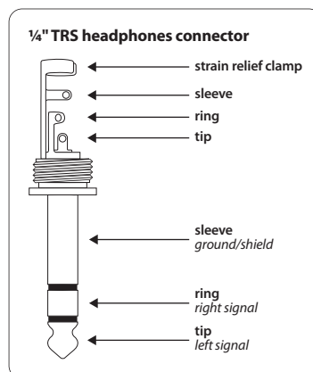
Рис. 4.2: Подключение стереоштекером наушников и стереоштекером для CD INPUT
