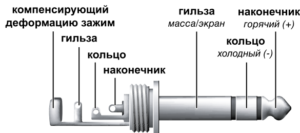
Рис. 4.2: 6,3-мм стереоштекер
