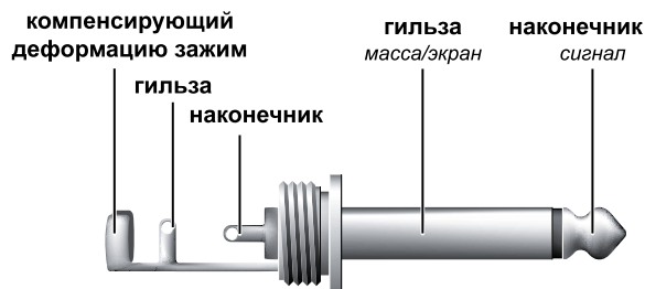
Рис. 4.1: 6,3-мм моноштекер
