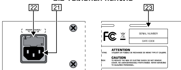
Рис. 2.2: Элементы управления на тыльной панели VIRTUBE
