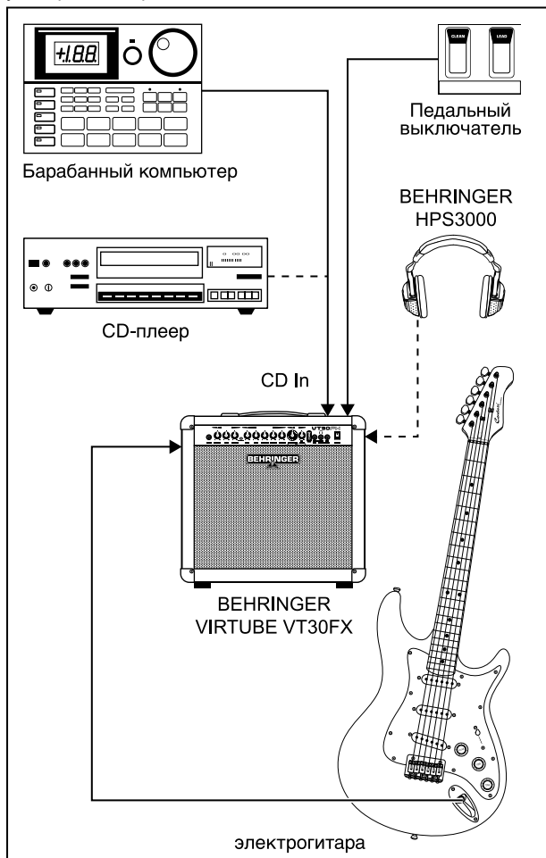
Рис. 3.1: Стандартный сетап с VT30FX
