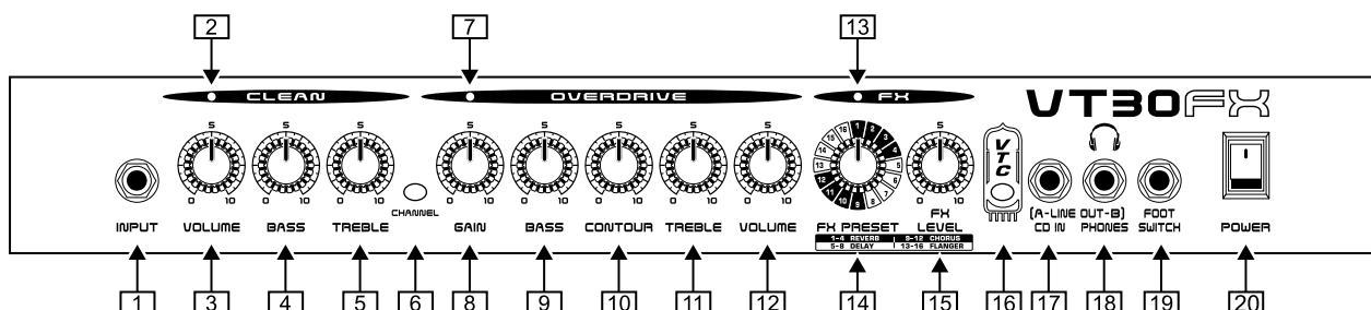
Рис. 2.1: Элементы управления на передней панели VIRTUBE
