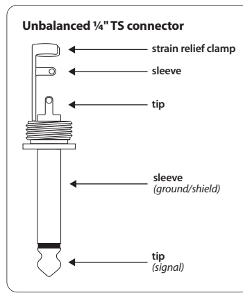
Рис. 3.3: 6,3-мм TS-штекер
