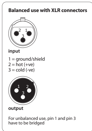
Рис. 3.1: Разъемы XLR
