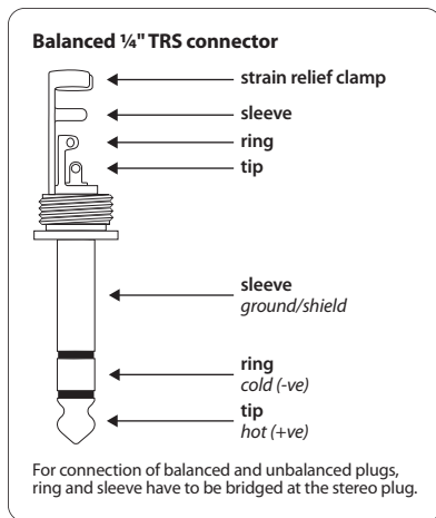
Рис. 3.2: 6,3-мм TRS-штекер
