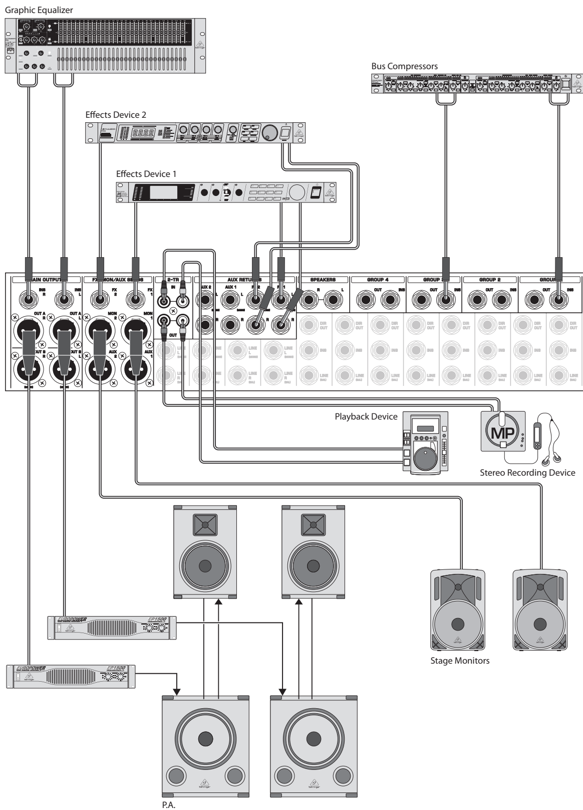
Рис. 2.1: Кабельное соединение каналов (выходы)
