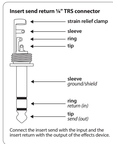
Рис. 3.4: Стереоштекер Insert-Send-Return
