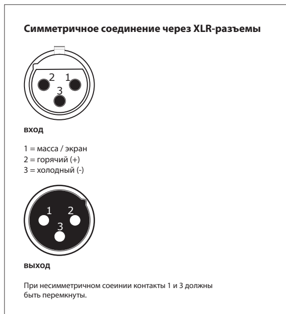
Rys. 3.1: Разъемы XLR
