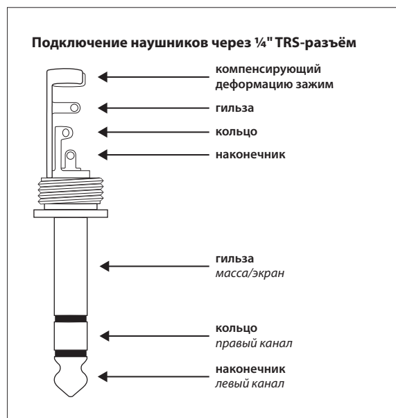
Рис. 3.5: Стереостекер наушников
