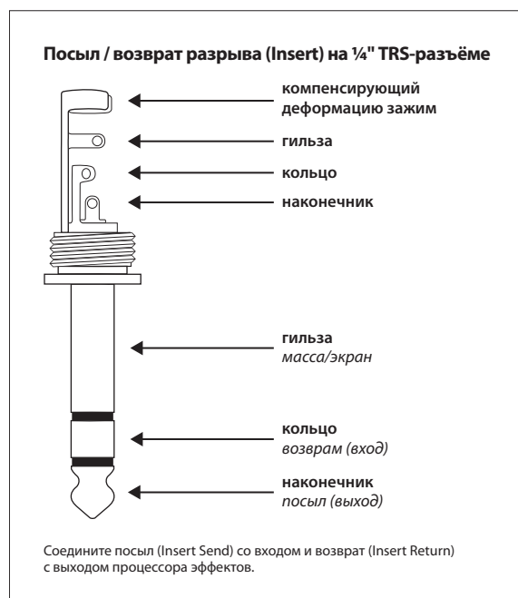
Рис. 3.4: Стереостекер Insert-Send-Return
