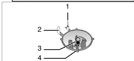
1 Устройство газ-контроля (в зависимости от модели)
