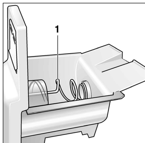
1 Подающий шнек
