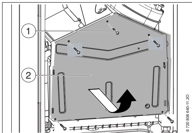
Рис. 38 Открытие горелки
