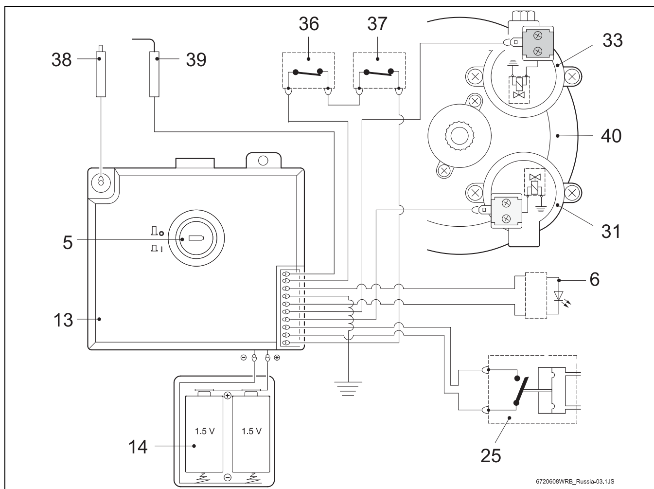
Рис 3 Электросхема
