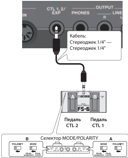
Подключение FS-6
