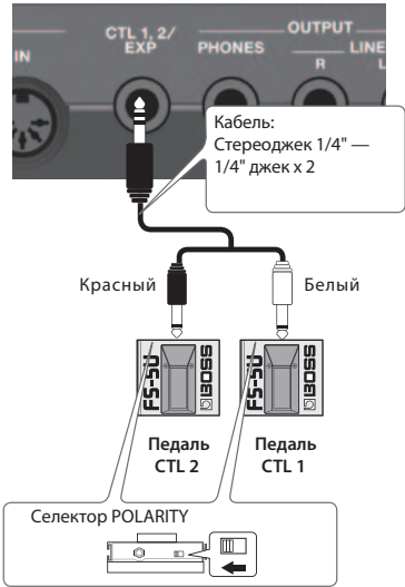
Подключение FS-5Us
