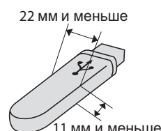
Флэш-накопитель USB
