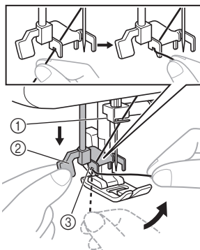
① Иглодержатель ② Рычажок нитевдевателя ③ Направляющая
