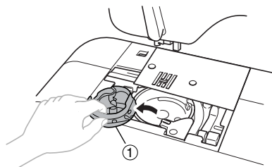
1 Подшпильник
